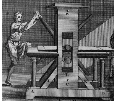
Görsel 2.11. Diderot'nun ansiklopedisindeki bir plakadan baskı haddeleme presinin detayı.
